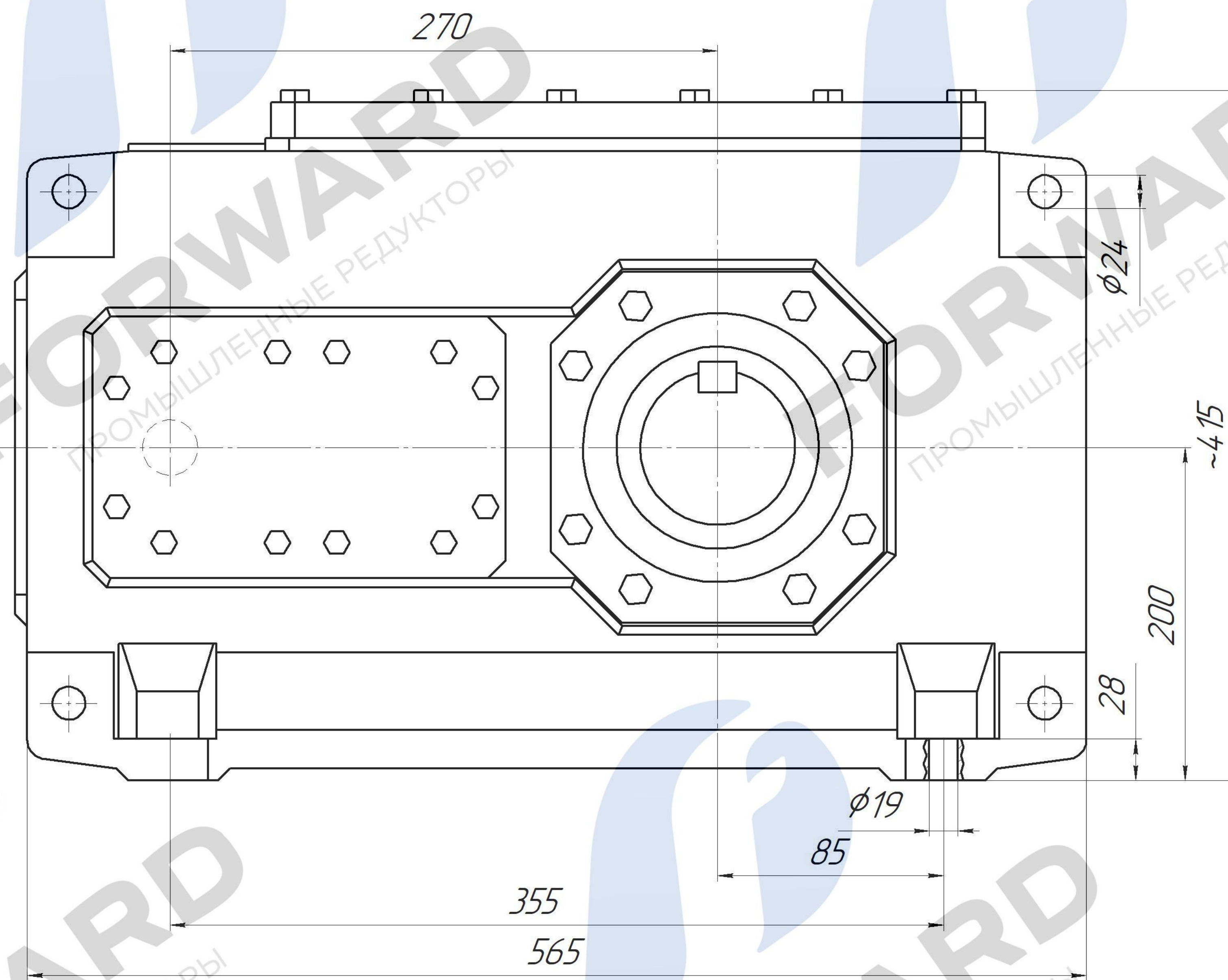
Вариант исполнения выходного вала
