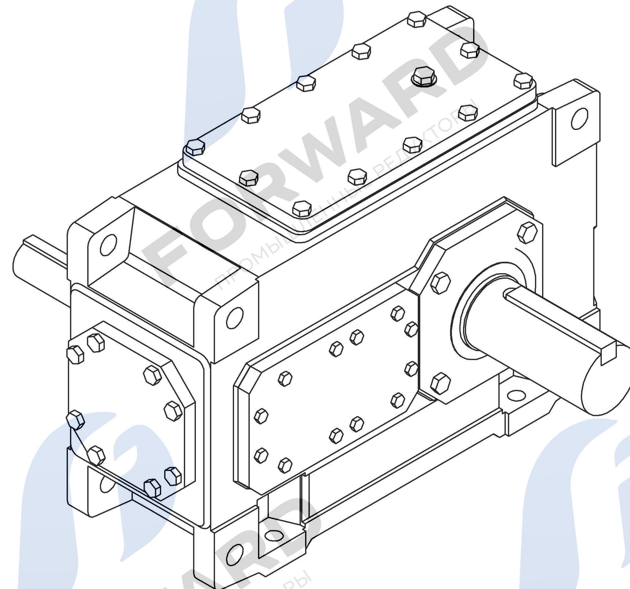
Вариант исполнения входного вала
