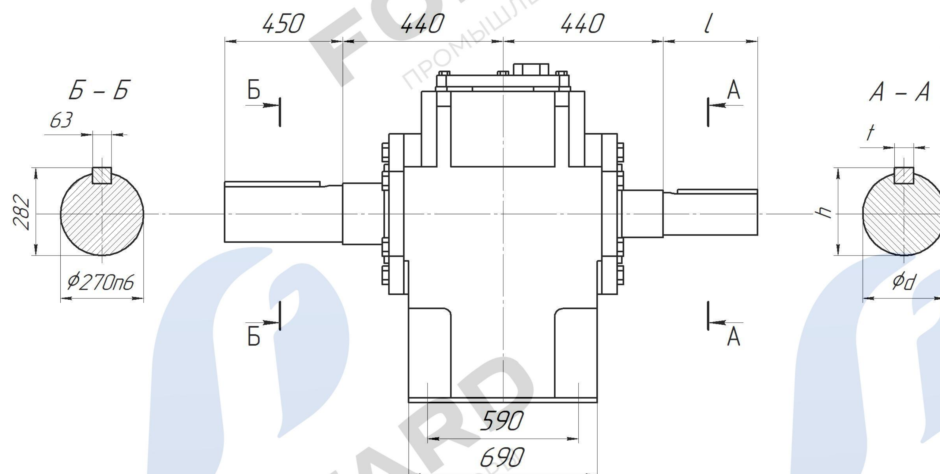
Цилиндрический вал
